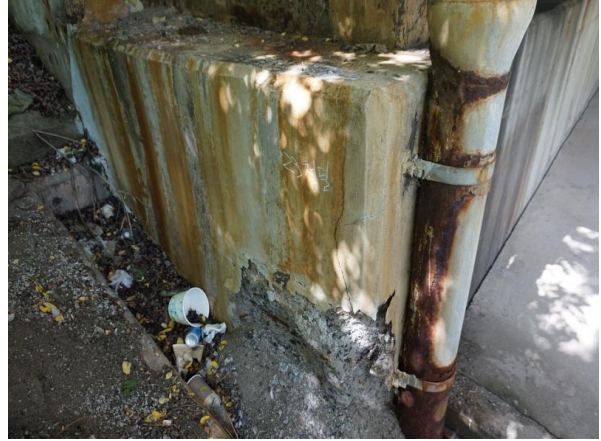
교대 박락 및 철근노출 A1(하절기)
