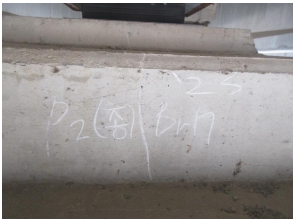
받침 콘크리트 균열(0.3mm미만) P2 A2-SH7
