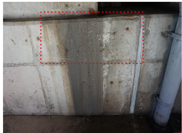
교대 박리 A1
